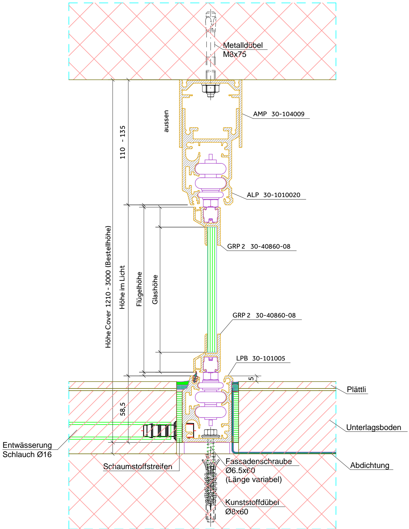
Bodendetail Schiene versenkt Entwässerung nach vorne mit Schlauch
