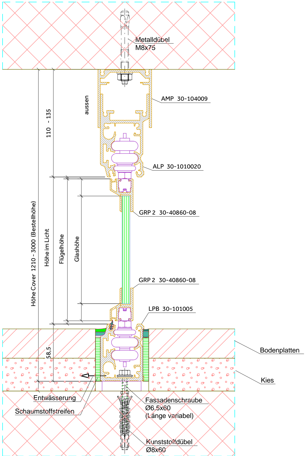
Bodendetail Schiene versenkt Entwässerung in Boden
