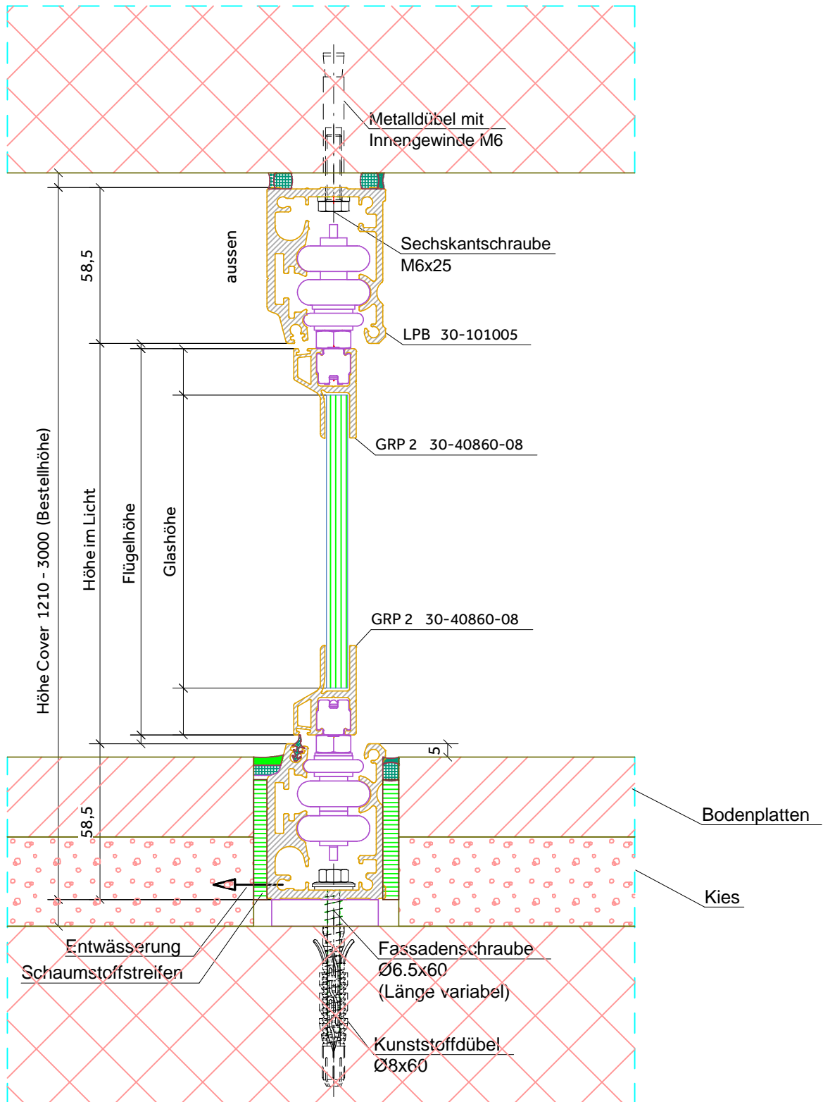
Bodendetail Schiene versenkt Entwässerung in Boden
