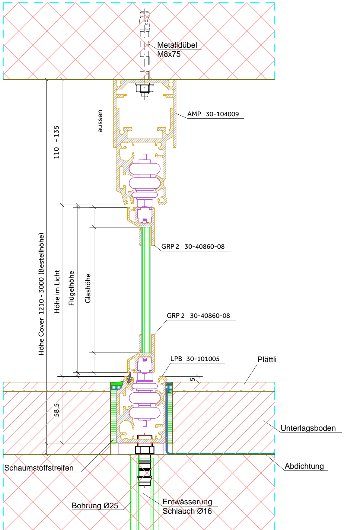
Bodendetail Schiene versenkt Entwässerung nach unten mit Schlauch
